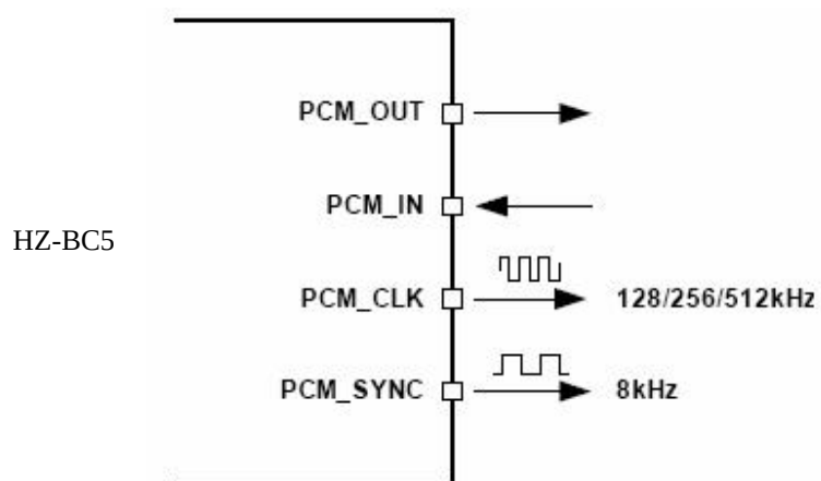
Figure 4:HZ-BC5 PCM 作为 MASTER 接口设计
