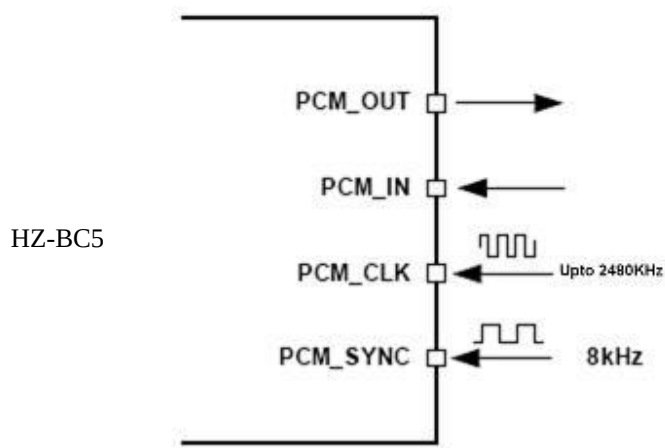
Figure 5:HZ-BC5 PCM 作为 SLAVE 接口设计
