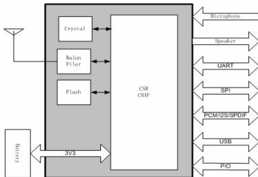
Figure 1: HZ-BC5 系统框图
